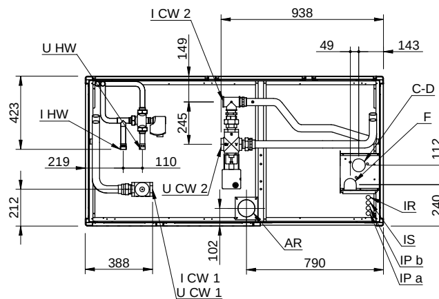
SEZIONE A-A
